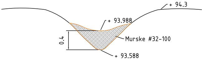
DETALJI A SUOTOPATO POIKKILEIKKAUS MALLIKUVA
